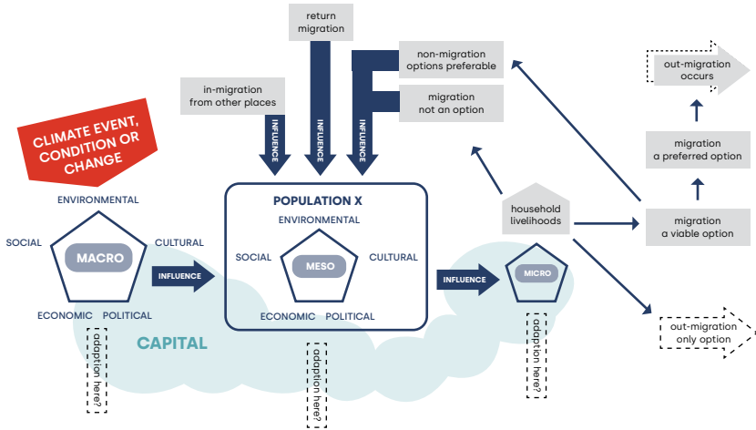
Figura 1 Rappresentazione concettuale della migrazione in un sistema adattativo (McLeman, 2014).
